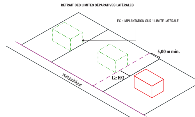
schéma n°4 DÉFINITION DU REcul PAR RAPPORT AUX LIMITES SÉPARATIVES
